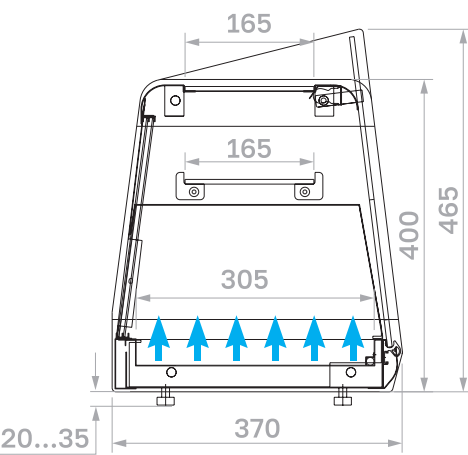
Статическое охлаждение
